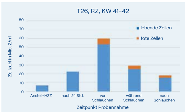
Hefezellzahlen über den Prozess
