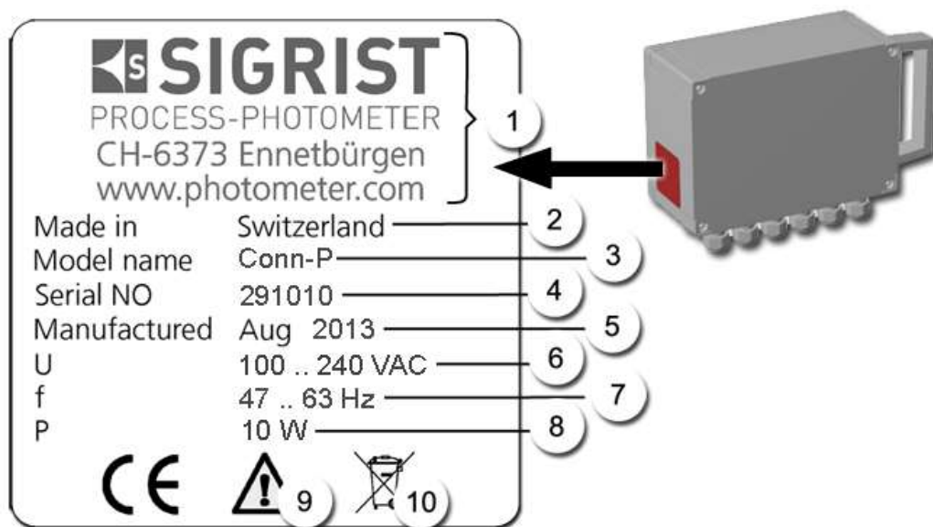
Abbildung 3: Typenschild Anschlussbox
